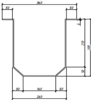
Секция водоотводного лотка (вид справа) М 1:5
