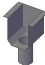
Общий вид конечной секции водоотводного лотка тип А М 1:10
